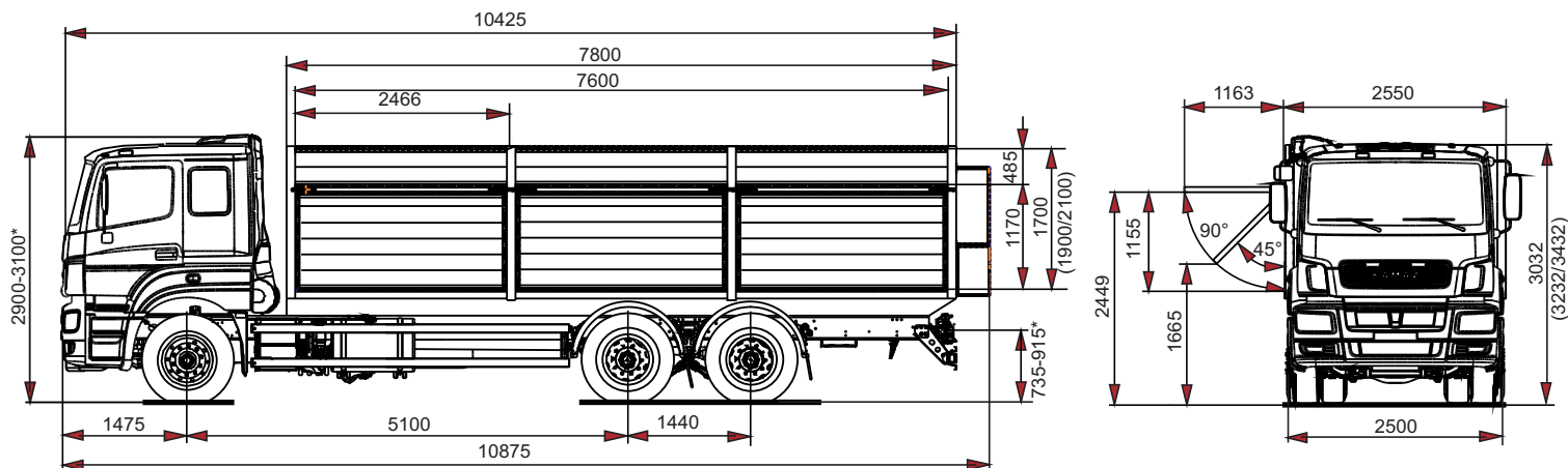
Размеры автомобиля снаряженной массы * - Размеры с учетом диапазона регулирования пневмоподвески
